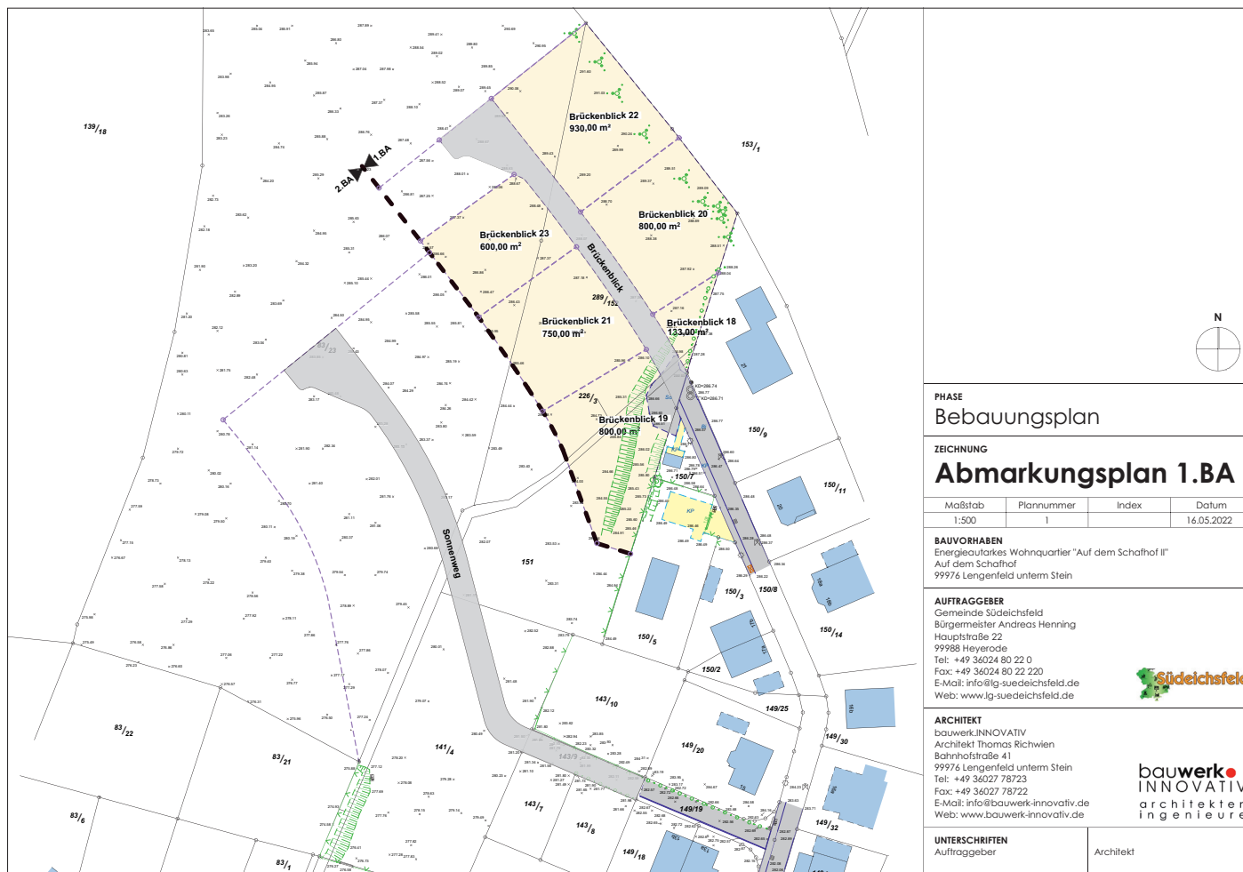
Abmarkungsplan Schafhof
